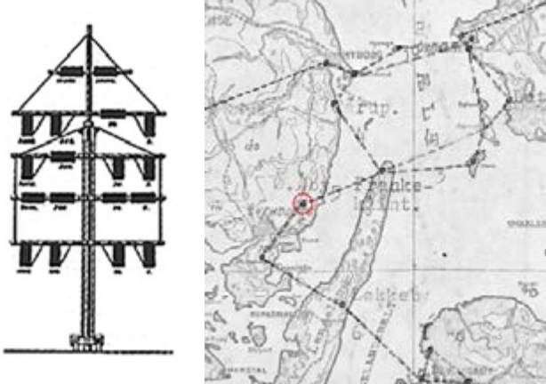
Tegning af den optiske telegrafstander + kort over telegrafsystemet omkring Storebælt. = Telegrafgården. (ÅRBOG FOR HISTORISK SAMFUND FOR SORØ AMT - 1972)
